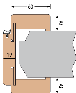
RK60 gerade
