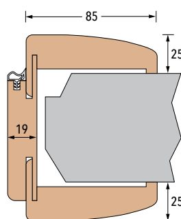
RK85 bombiert
