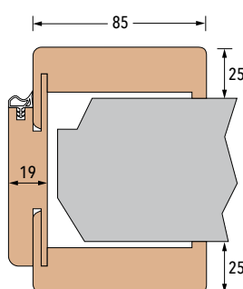
RK85 gerade
